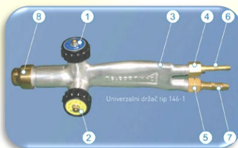
Slika 21; univerzalno držalo
